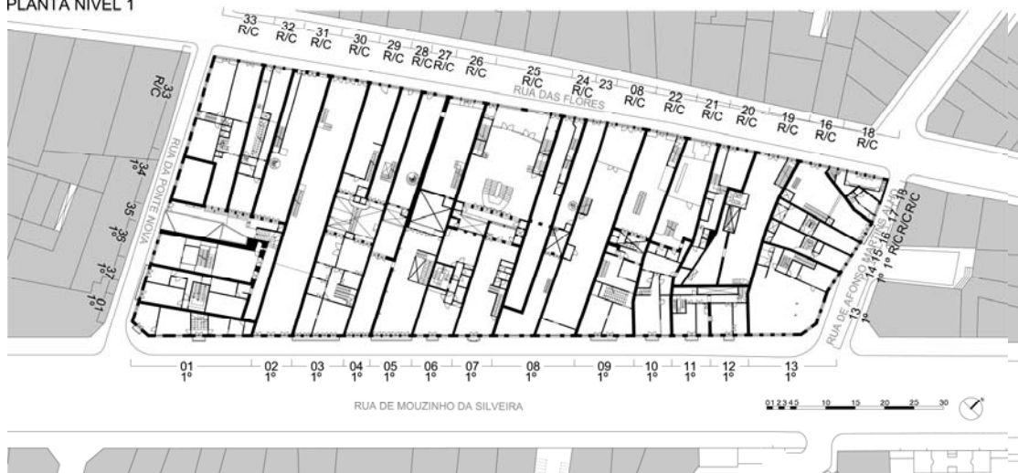
PLANTA NÍVEL 1
